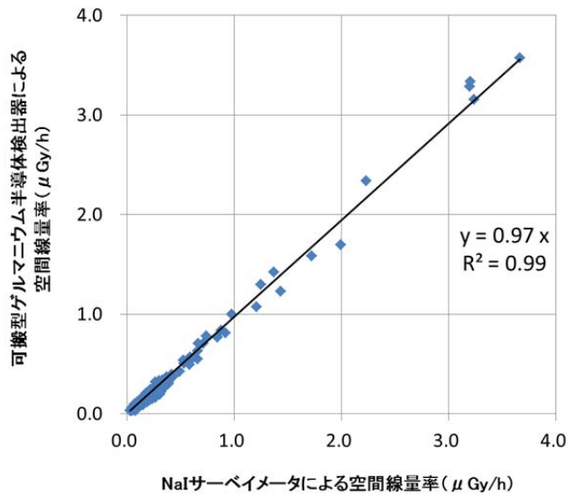
図-2 可搬型ゲルマニウム半導体検出器による in-situ 測定の結果を基に求められた空間線量率 ( \mu\text{Gy/h} ) とサーベイメータによる空間線量率 ( \mu\text{Gy/h} ) の相関 (平成 27 年 8 月 24 日～10 月 7 日に測定)
