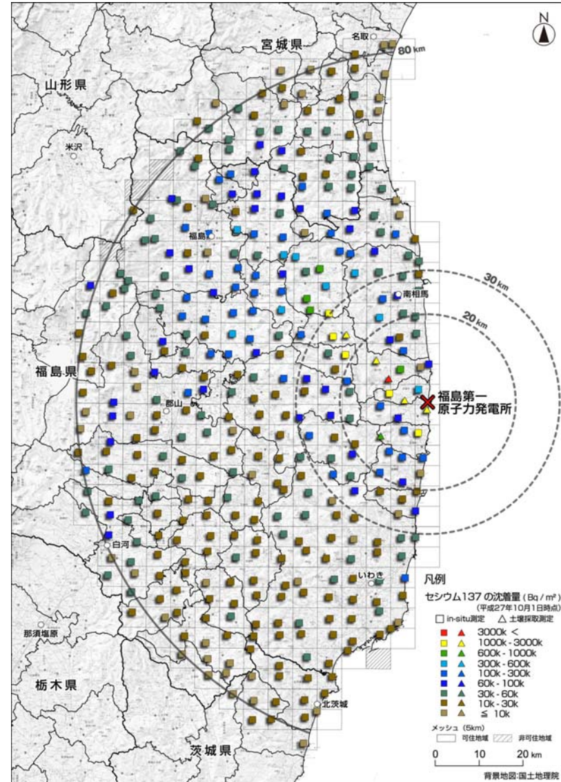
図-3 可搬型ゲルマニウム半導体検出器による in-situ 測定等を用いた放射性セシウムの沈着量を記したマップ (平成27年10月1日時点: 緩衝深度 \beta = 2.95 \text{ g/cm}^2 を用いた解析結果。左図がセシウム134、右図がセシウム137)
